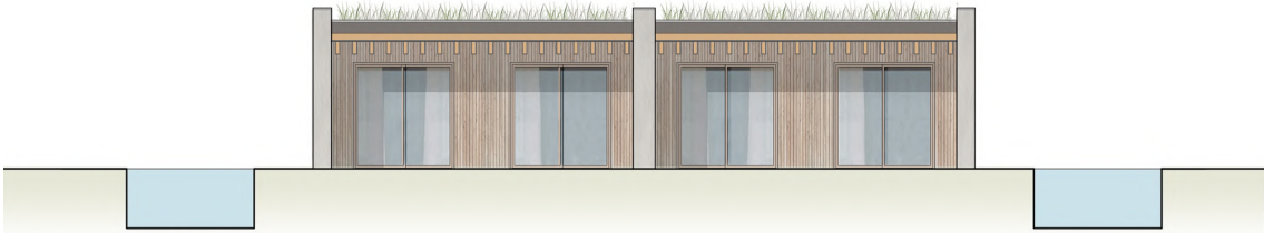
PROSPETTO FRONTALE
