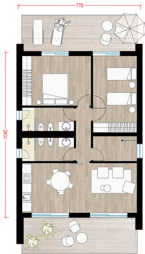
UNITA' SINGOLA
